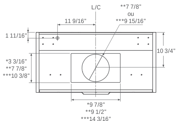
Dimensions – conduit et électricité
