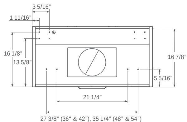
Dimensions d'installation
