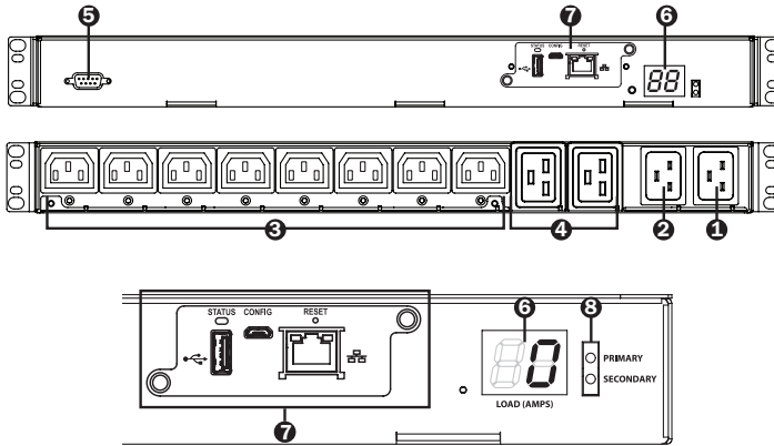
PDUMH20HVAT, PDUMH20HVATNET
