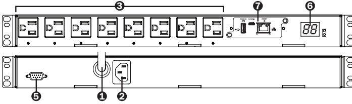
PDUMH15HVAT, PDUMH15HVATNET
