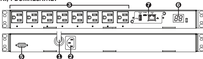
PDUMH15HVAT, PDUMH15HVATNET
