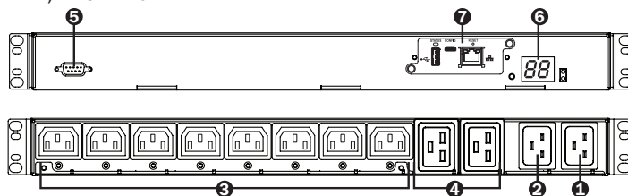
PDUMH20HVAT, PDUMH20HVATNET
