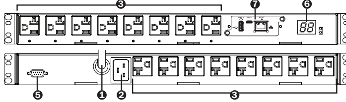
PDUMH20HVAT, PDUMH20HVATNET
