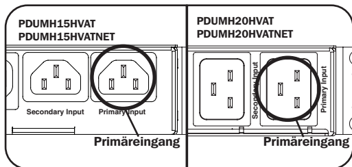
Primäreingang (208 - 240 V-Modelle)
