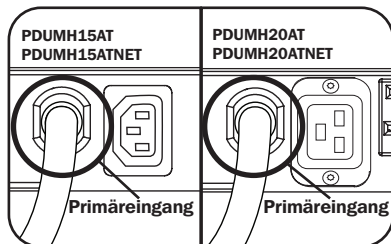
Primäreingang (120 V-Modelle)
