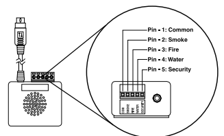
Рисунок 3: Подключение к EnviroSense устройств Contact Closure [закрывание контактов]
