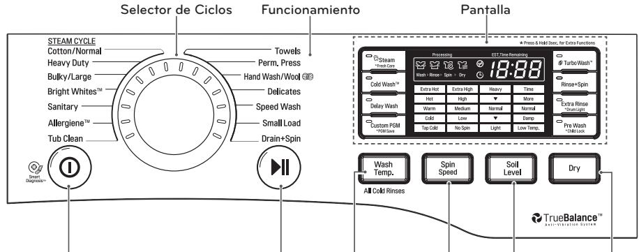
Botón de Encendido Funcionamiento Botón de Inicio/Pausa Botón de Selección de Temperatura de Agua Botón de Selección de Velocidad de Centrifugado Botón de Selección de Nivel de Suciedad Botón de Selección de Nivel de Suciedad SECADO Botón de Selección de Nivel de Suciedad
