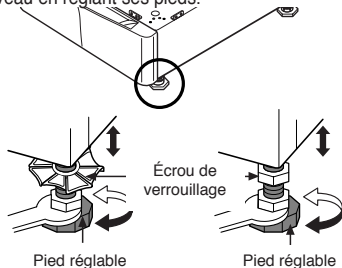
Pied réglable
