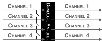
Abb. 4.6.1 Vier Kanäle ohne Eingangs-Routing
